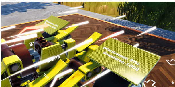
Aktive Aerodynamiksimulation über den Downforce-Flügeln.
